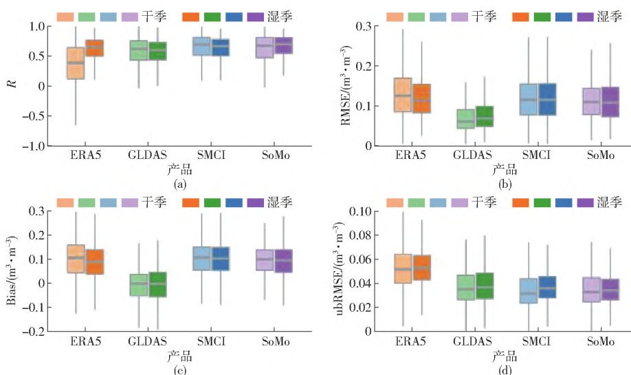
图9 黄土高原干湿季4种产品土壤湿度精度评价结果
