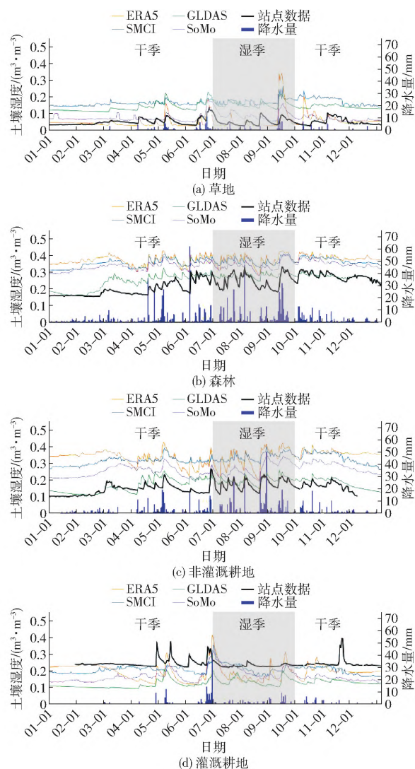
图 10 2019 年黄土高原不同土地覆盖类型下代表性站点土壤湿度时间序列曲线
