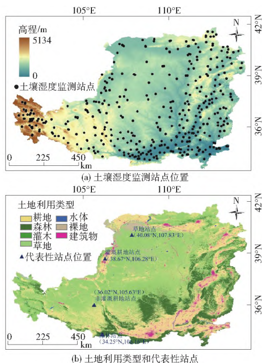
图1 黄土高原土壤湿度监测站点位置与土地利用类型和代表性站点空间分布
