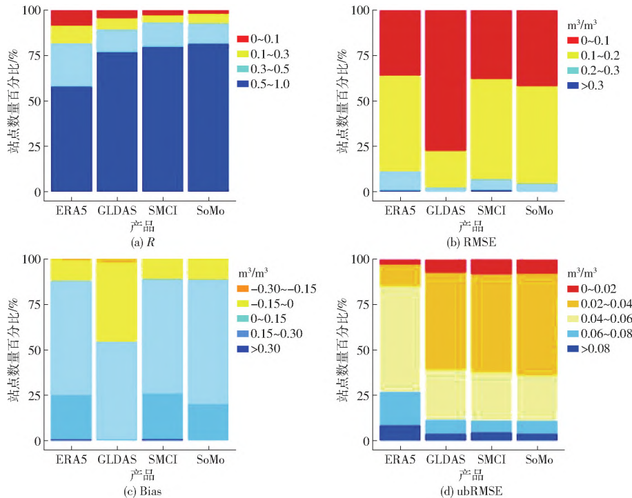
图7 黄土高原土壤湿度不同精度观测站点数量百分比
