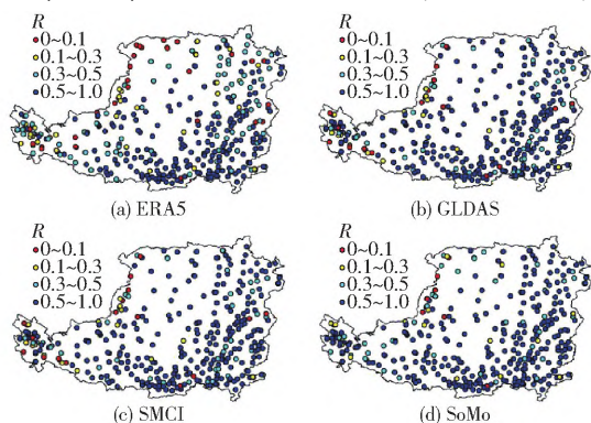
图3 不同产品土壤湿度与站点实测值间相关系数空间分布
