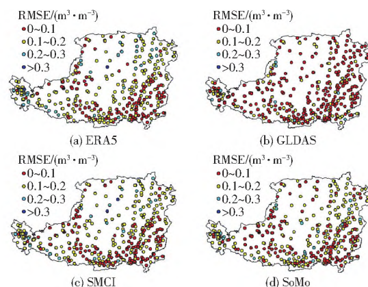
图4 不同产品土壤湿度与站点实测值间均方根误差空间分布
