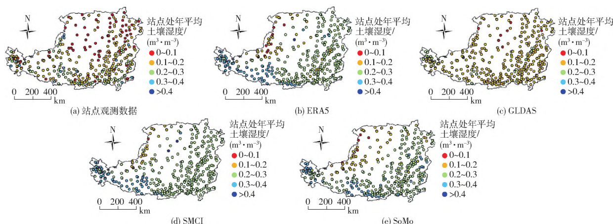
图2 黄土高原各站点 2016—2019 年平均土壤湿度
