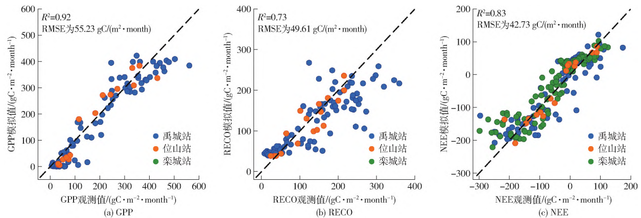
图3 禹城站、位山站和栾城站月尺度 GPP、RECO、NEE 的模型模拟精度验证
