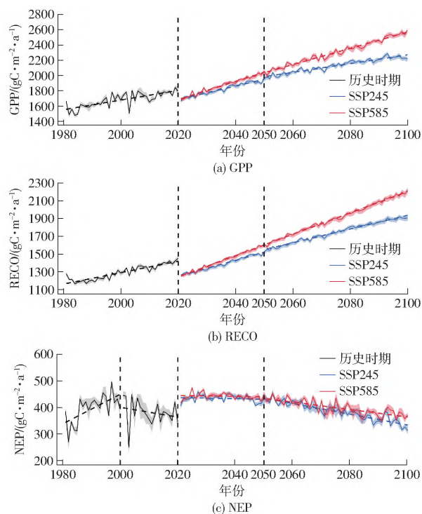
图4 黄淮海平原麦玉轮作区 1981—2100 年 GPP、RECO、NEP 的年际时间变化趋势
