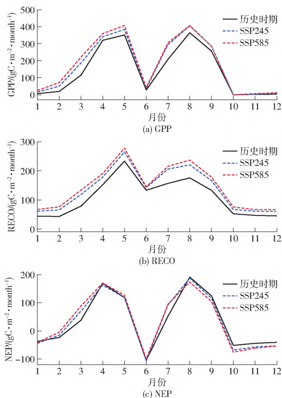
图5 历史时期(1981—2020年)和未来(2021—2100年)两种情景(SSP245 和 SSP585)下黄淮海平原麦玉轮作区 GPP、RECO、NEP 的年内变化
