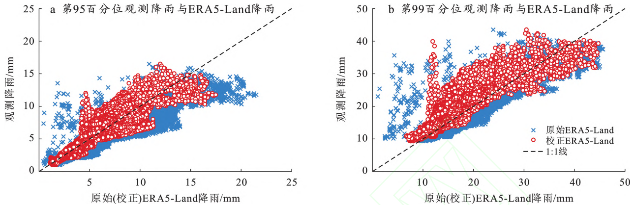
图 4 第 95 分位和第 99 分位校正前后降雨量的散点图
