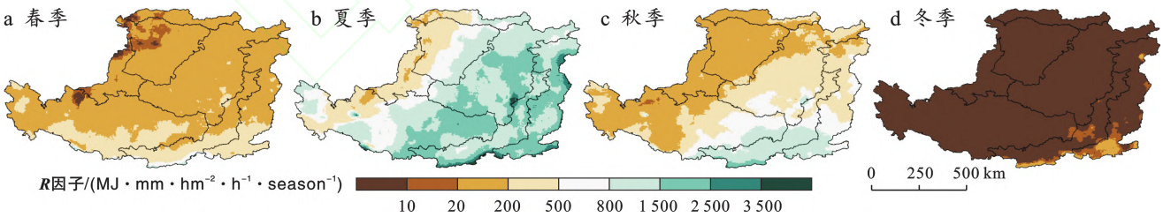
图 7 黄土高原 2001—2024 年校正后 ERA5-Land 降雨驱动的季节性 R 因子空间分布
