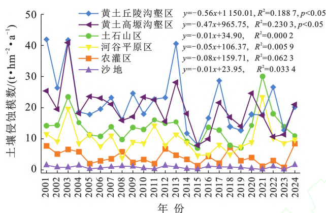
图9 黄土高原生态分区2001—2024年土壤侵蚀模数年际变化
