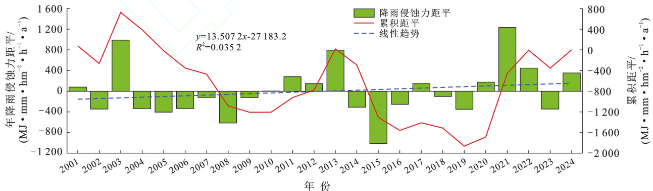
图 5 黄土高原 2001—2024 年降雨侵蚀力变化特征
